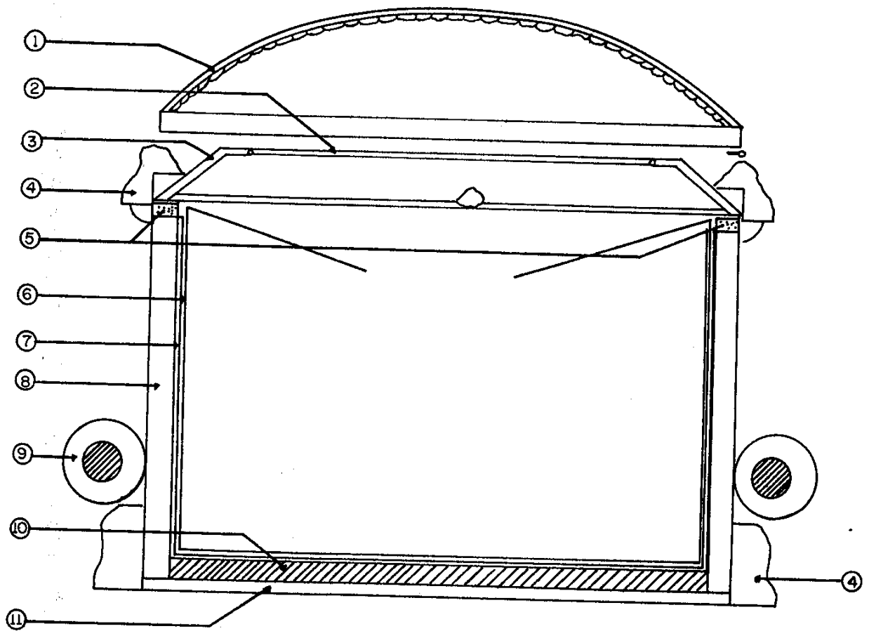
CORTE A-A Esc: 1:5
