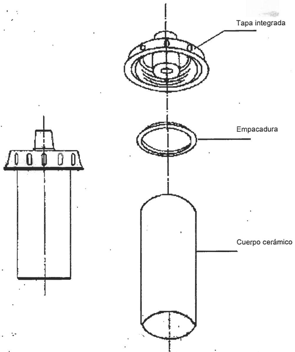
Figura 2. Elemento purificador ciego con tapa (Tipo B)
