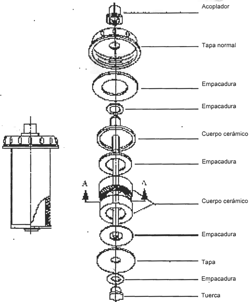
Figura 5. Elemento purificador con tapa normal (Tipo E)
