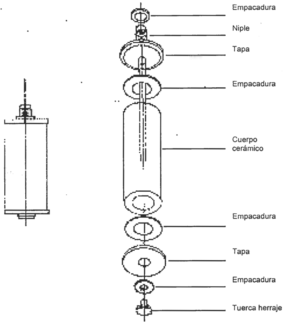
Figura 3. Elemento purificador con herraje (Tipo C)
