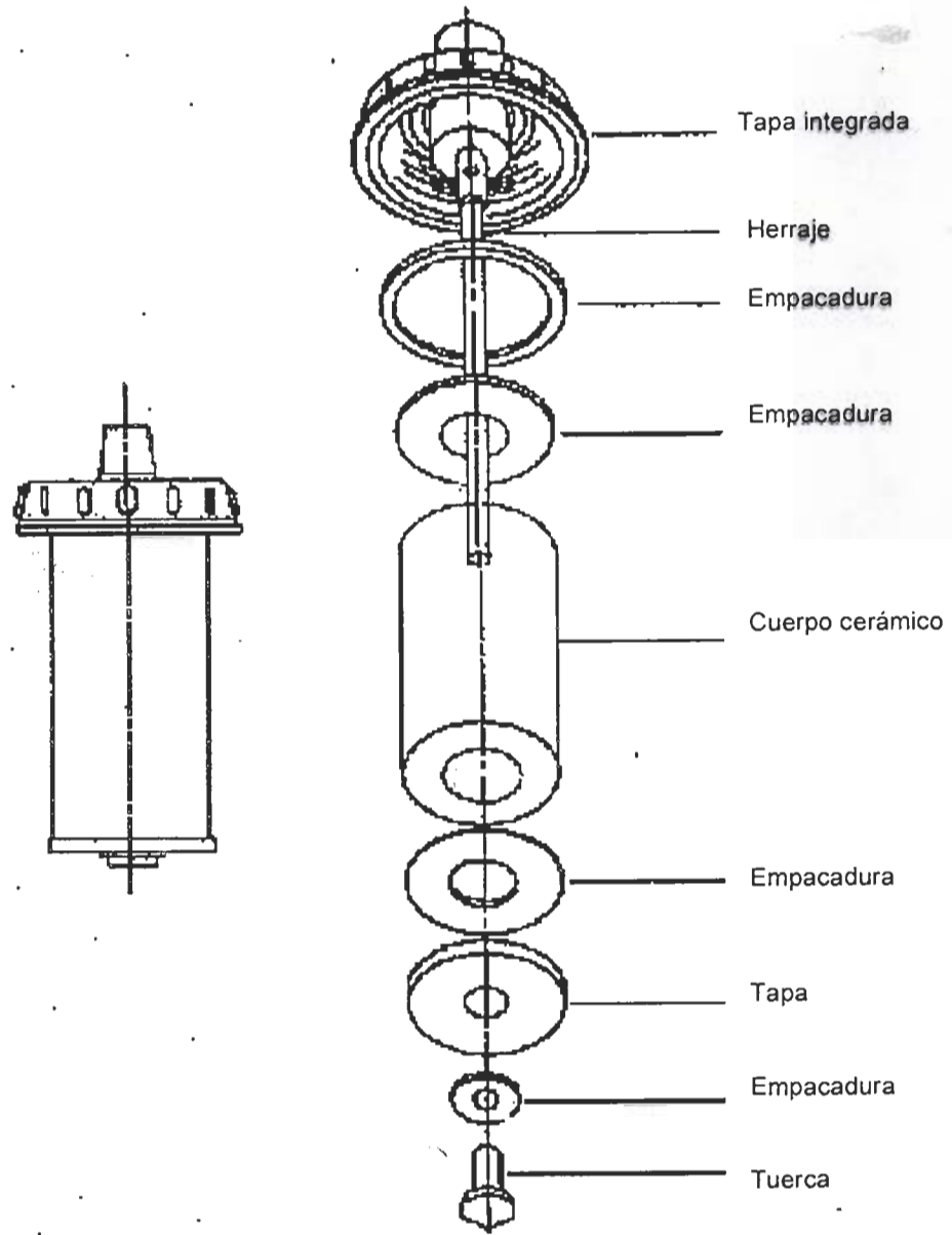
Figura 4. Elemento purificador con herraje integrado (Tipo D)
